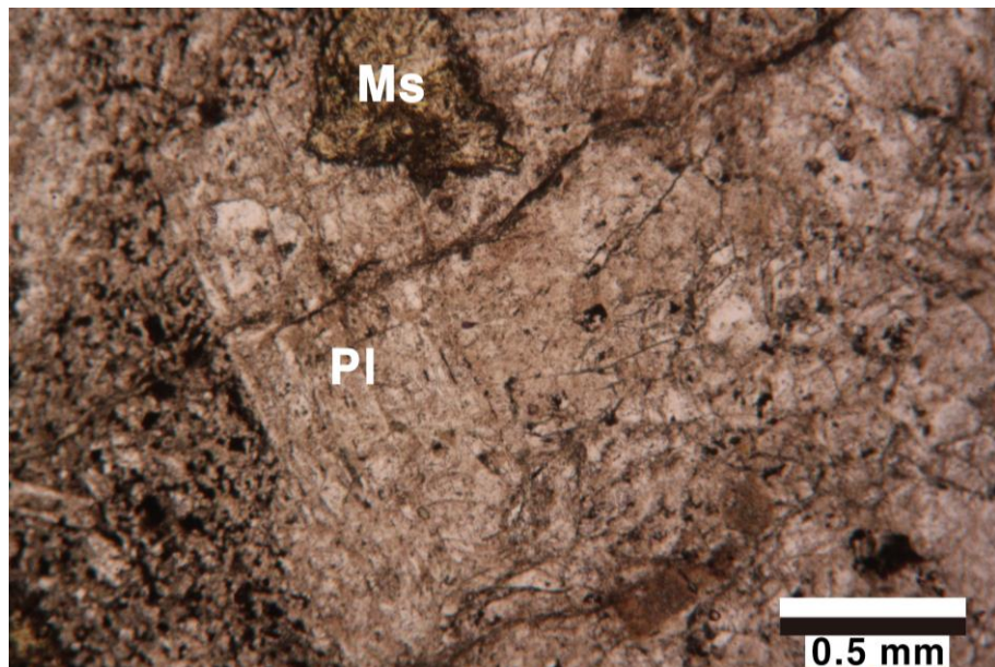
Bt: biotite(흑운모), Ms: muscovite(백운모), Pl: plagioclase(사장석).
